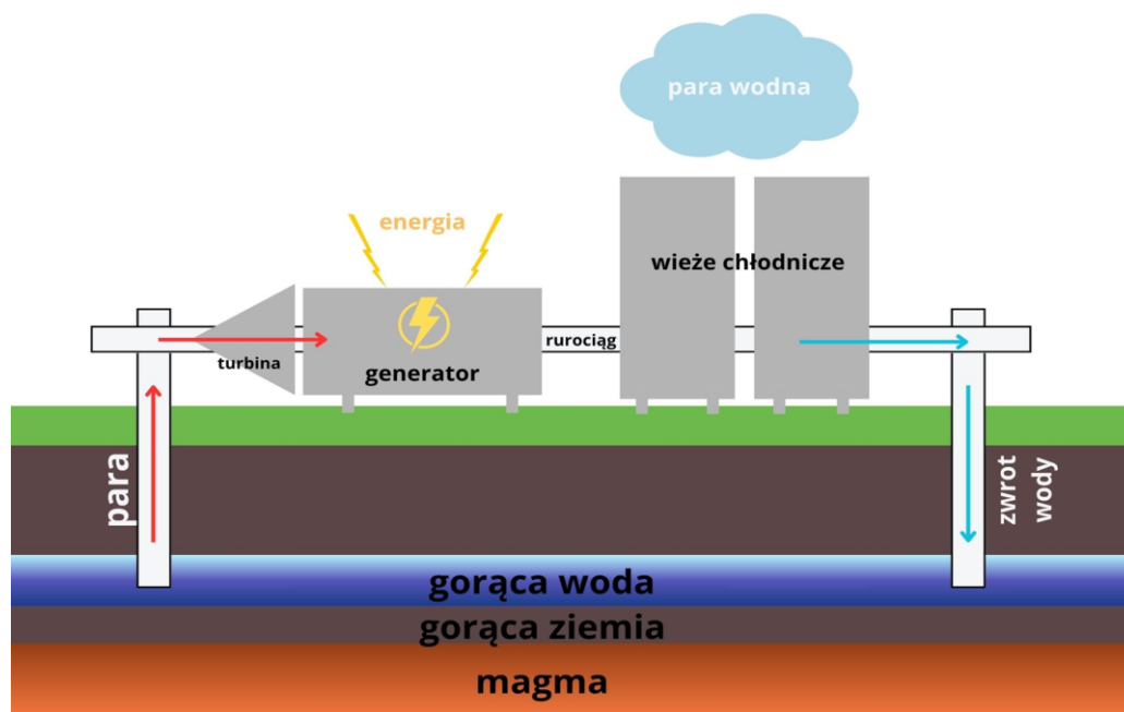
Schemat elektrowni geotermalnej
